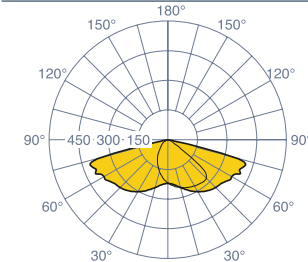
Thor S - montage en top
