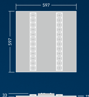
OMEGA MODULINE 600 X 600
