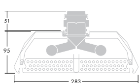
T8 vit eller perforerad stomme med vitt eller perforerat bländskydd, 2-rörs
