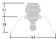
T8 vit reflektor 1- rörs
