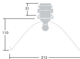
T8 aluminiumreflektor med smal ljusfördelning 1-rörs
