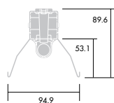
1-rörs med symmetrisk reflektor
