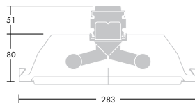
T8 vit reflektor med vitt bländskydd 2- rörs
