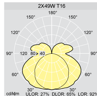
2-rörs med symmetrisk reflektor
