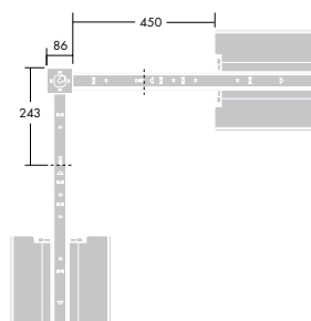
Skenkopplingar (T-CX)
