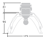
T8 symmetrisk ljusfördelning 1-rörs
