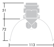
T5 aluminiumreflektor med bred ljusfördelning 1-2 rörs
