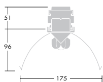
T5 aluminiumreflektor med smal ljusfördelning 1-2 rörs
