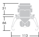
T5 bred ljusfördelning 1-2 rörs
