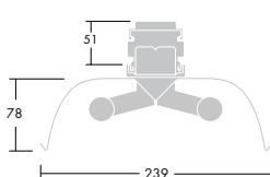
T8 aluminiumreflektor med bred ljusfördelning 2-rörs
