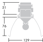
T8 aluminiumreflektor med bred ljusfördelning 1-rörs
