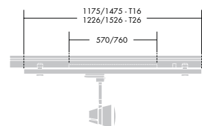
Spotlightmodul
