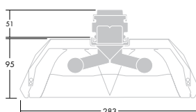
T8 Matt bländskydd, 2-rörs
