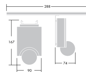
modul med närvaro-detektor
