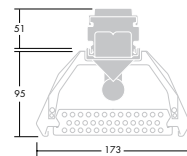
T8 vit eller perforerad stomme med vitt eller perforerat bländskydd, 1-rörs
