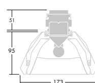
T8 Matt bländskydd, 1-rörs
