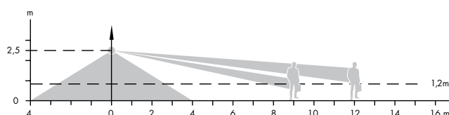
Närvarodetektorns detekteringsområde, upp till 16 m avstånd
