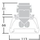
T5 vitt bländskydd, 1-rörs
