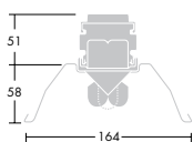
T5 vit reflektor, 1- eller 2-rörs
