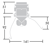
T5 aluminiumreflektor, väggreflektor (wall washer) 1-2 rörs
