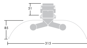
T8 aluminiumreflektor med smal ljusfördelning 2-rörs
