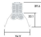
2-rörs med symmetrisk reflektor
