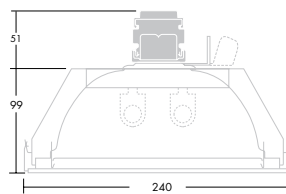
Industrivariant IP60
