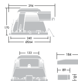
Cruz 240 H med separat driftdon (HFD)
