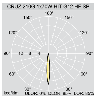
Cruz 210G med externt drifdon (HIT/HST)
