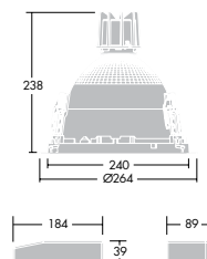
Cruz 240 V med separat driftdon (HST)
