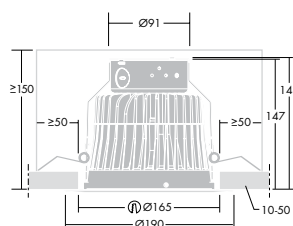
infälld 12W
