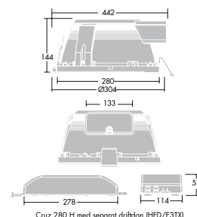
Cruz 280 H med separat driftdon (HFD/E3TX)
