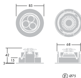
Mellan DL
