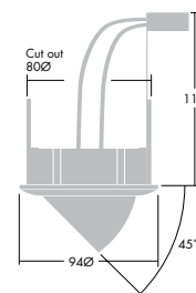
Ställbar +/- 0 - 45°
