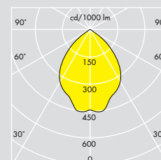
AL357 vertikal HF Ljuskälla: 1 x 42W TC-TEL ULOR: 0% DLOR: 74% LOR: 74%
