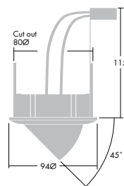
Ställbar +/- 45°
