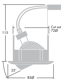
Ställbar +/- 0-25°
