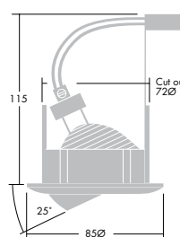
Ställbar +/- 0 - 25°
