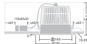
infälld 18W
