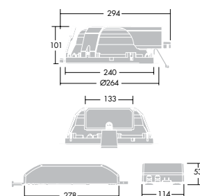
Cruz 240 HL med separat driftdon (HFD/E3TX)
